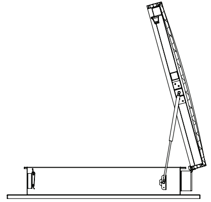
SECÇÃO A-A
