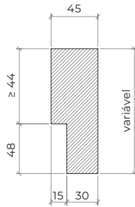
aro modificado | montagem em parede de gesso cartonado | fixação com espuma expansível em pórtico metálico
