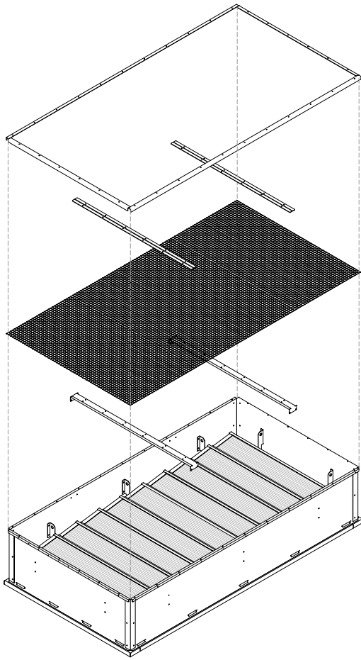
ESQUEMA DE MONTAGEM
