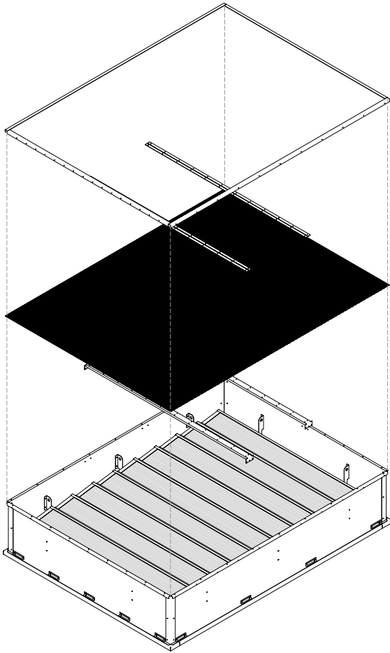
ESQUEMA DE MONTAGEM
